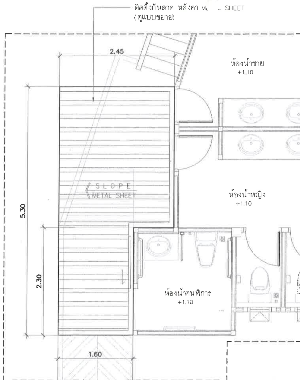
แบบแปลนติดตั้งหลังคาติดตั้งสาด
