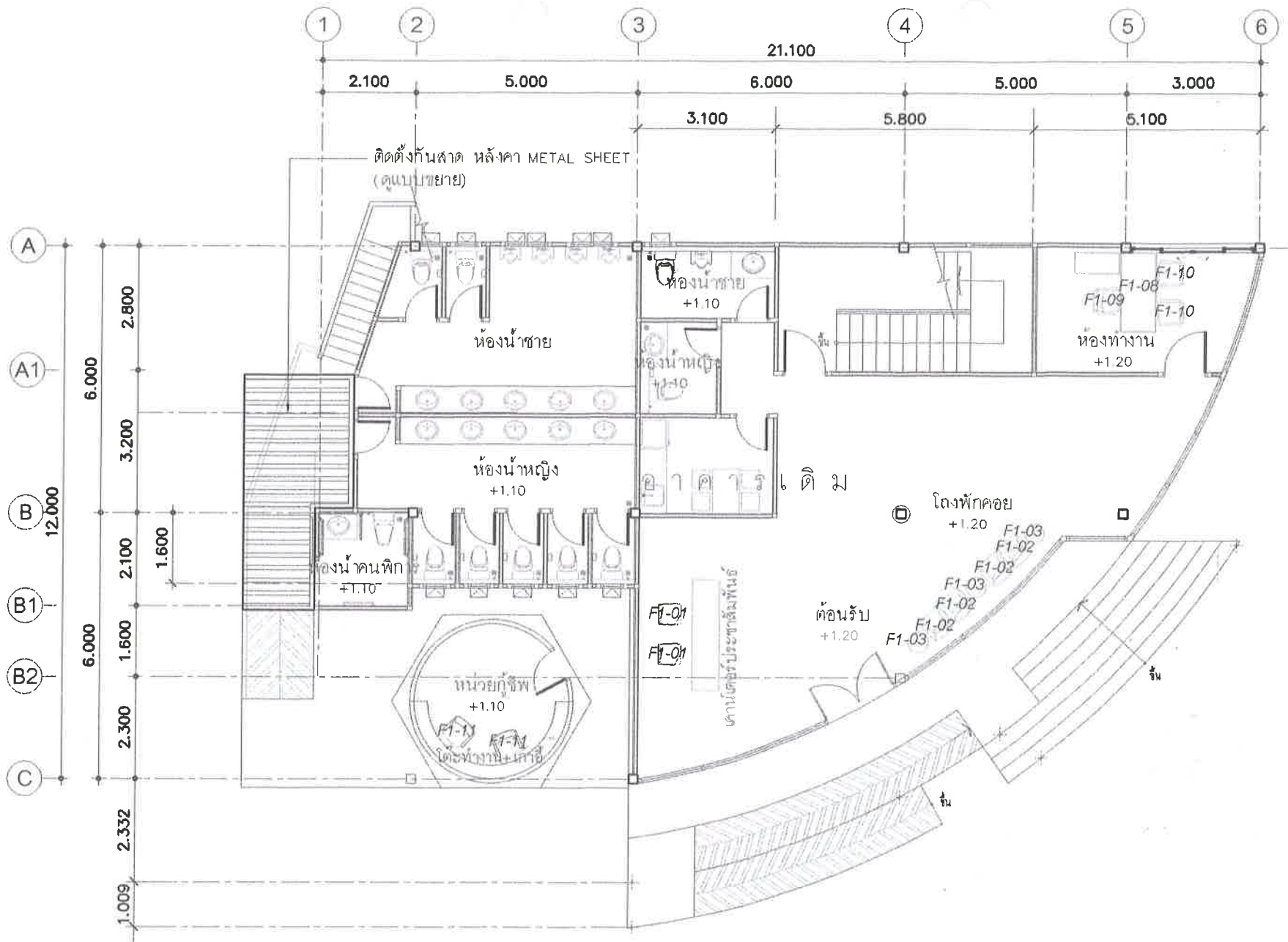
แบบแปลนงานตกแต่งภายใน 2 ชั้นล่าง SCALE 1:125
