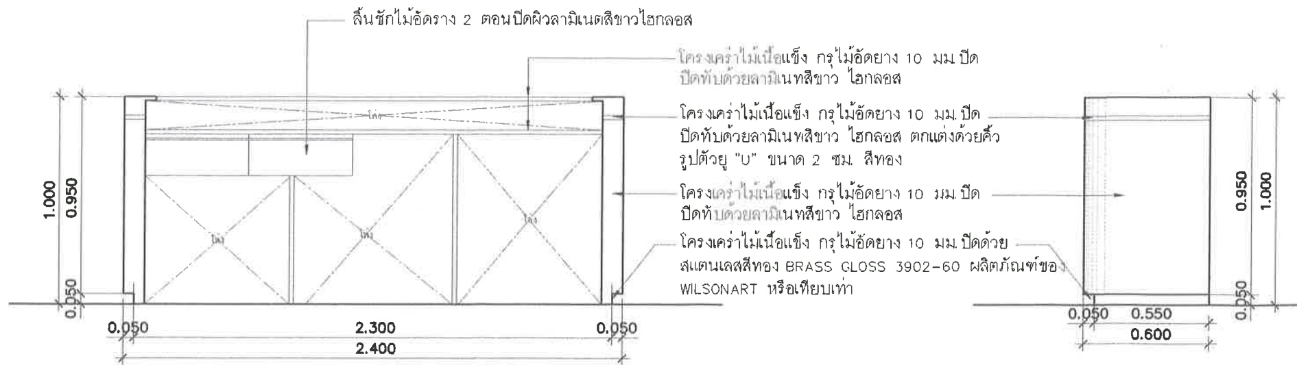
แบบรูปด้านขวา SCALE 1:25
