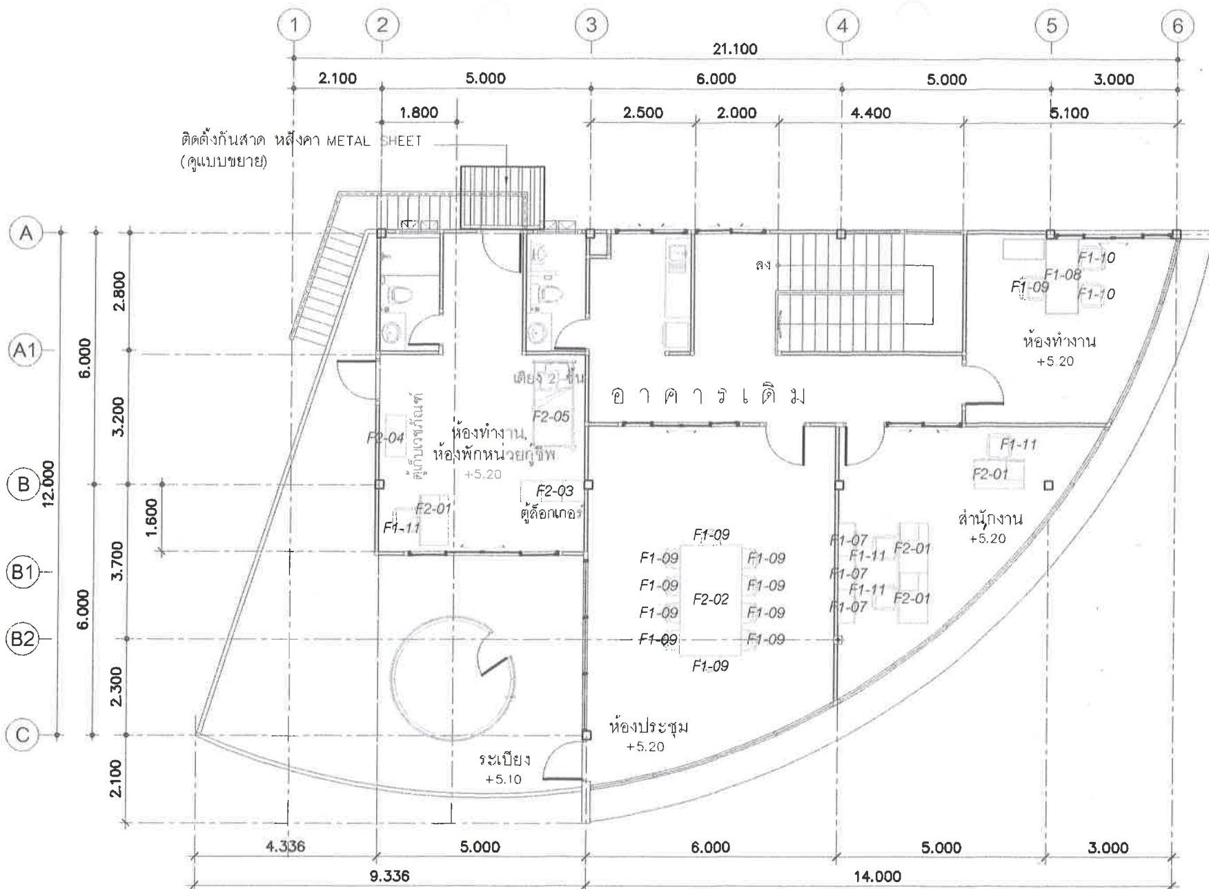
แบบแปลนงานตกแต่งภายใน ชั้น 2 SCALE 1 : 125
