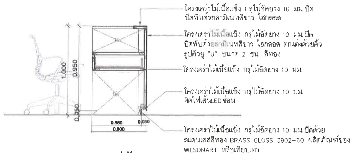
แบบขยายเคาน์เตอร์ประชาสัมพันธ์ SCALE 1:25
