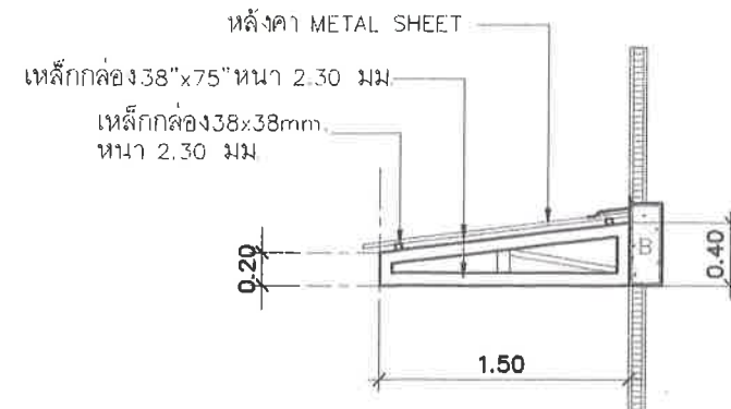
รูปตัด SCALE 1 : 50
