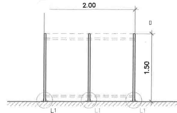
แบบแปลนโครงหลังคาถัดสาด SCALE 1 : 50
