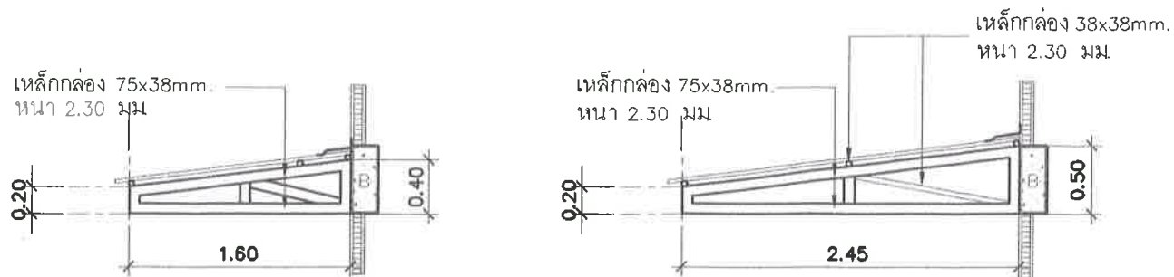
รูปตัด SCALE 1 : 50
